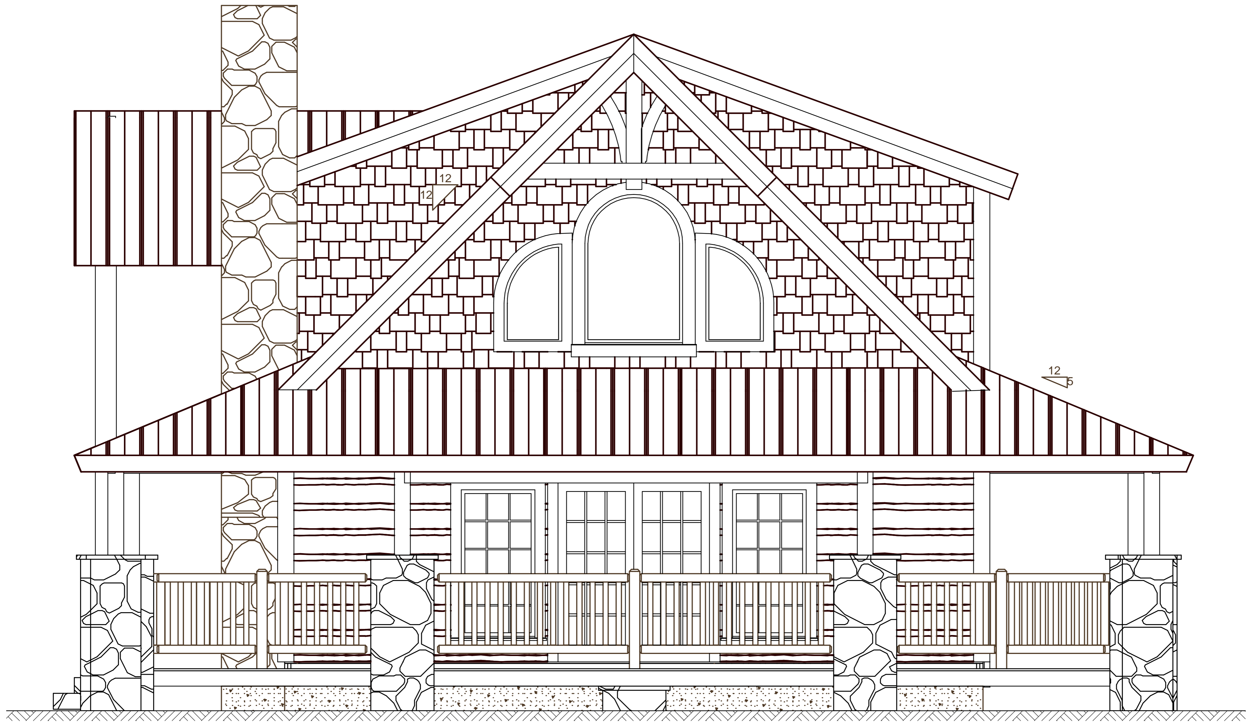
RIGHT ELEVATION
